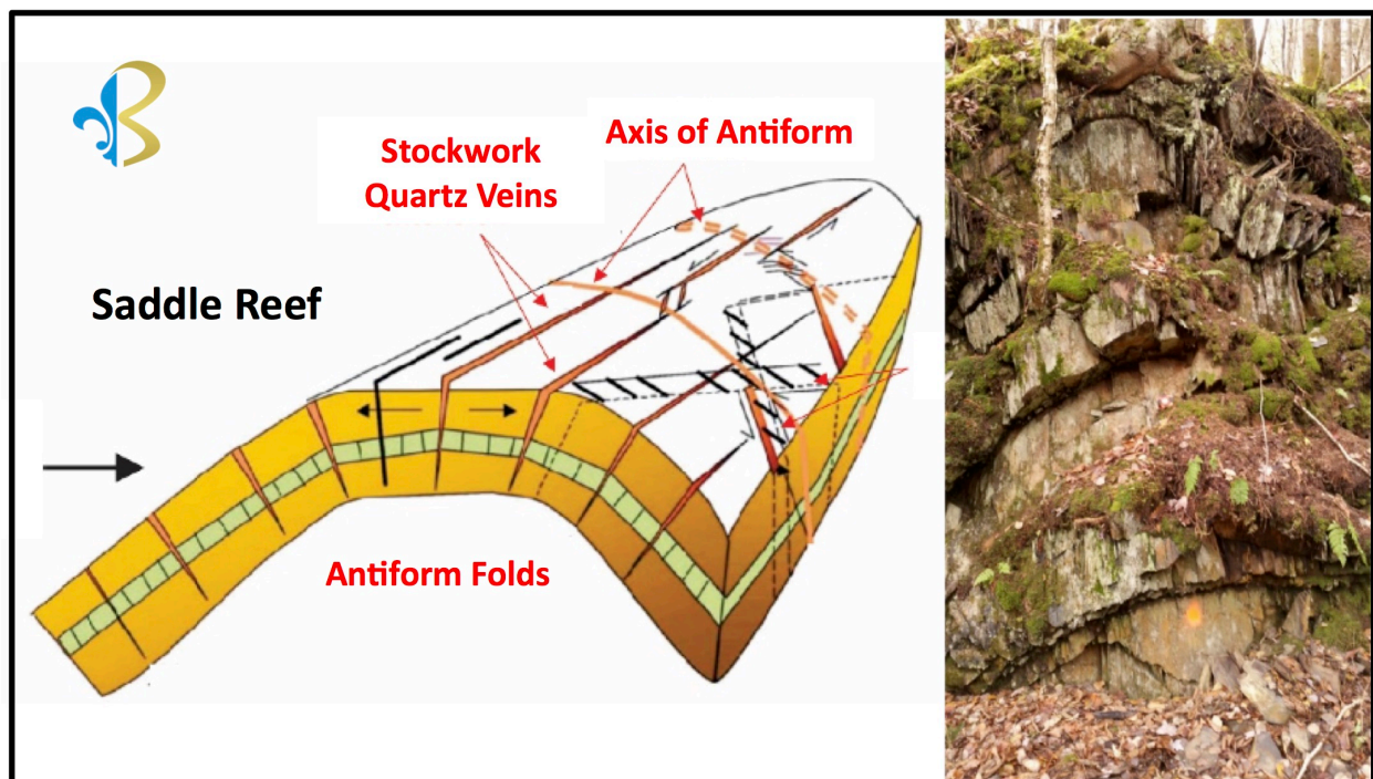
Image 1 : Diagramme en coupe transversale des plis antiformes. A droite, Plis Antiformes coupés le long du Ruisseau Giroux dans le Rang Delery
