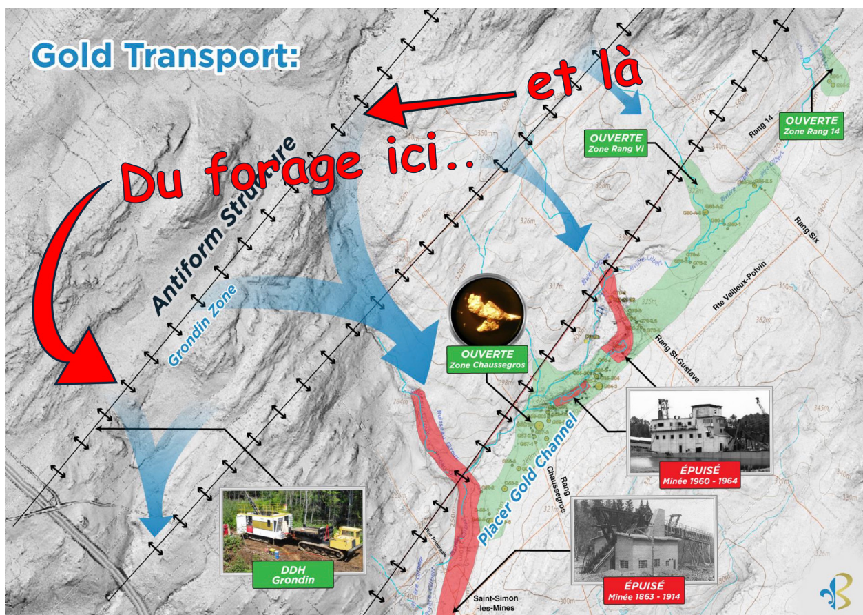
Image : Flux de transport de l'or depuis les structures anti-forme vers le canal Placer
