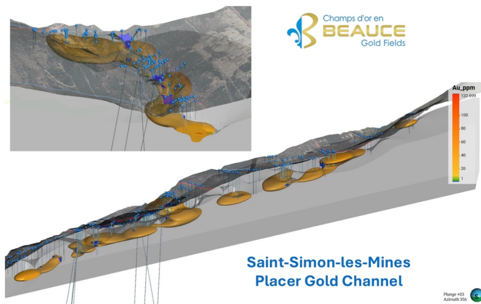
Image : Vue 3D du canal aurifère placérien, en médaillon, coupe transversale au rang Chaussegros
